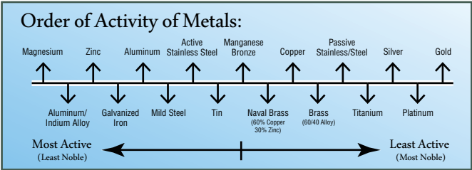
Figure 11-1: Sacrificial Anodes
